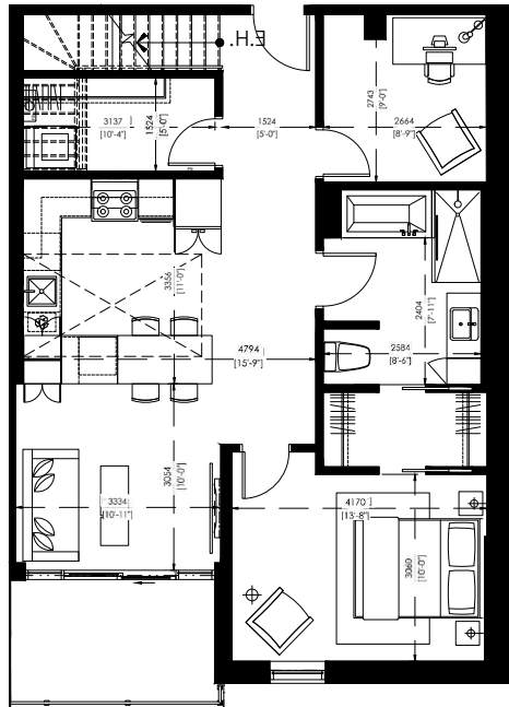
Étage principal
